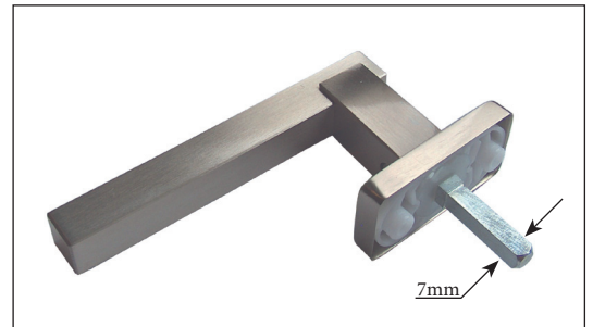
895 CW/325 ΠΟΜΟΛΟ Europa (μικρό) LEVER HANDLE Europa (short)
