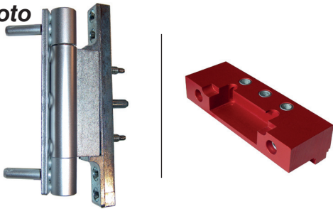
190588 ΡΥΘΜΙΖΟΜΕΝΟΣ ΜΕΝΤΕΣΕΣ ΠΟΡΤΑΣ ADJUSTABLE DOOR HINGE 1169409 ΣΤΑΜΠΟ ΠΟΡΤΑΣ ΓΙΑ ΤΟΝ ΜΕΝΤΕΣΣΕ 190588 DOOR PIERING ACCESSORY FOR 190588 HINGE
