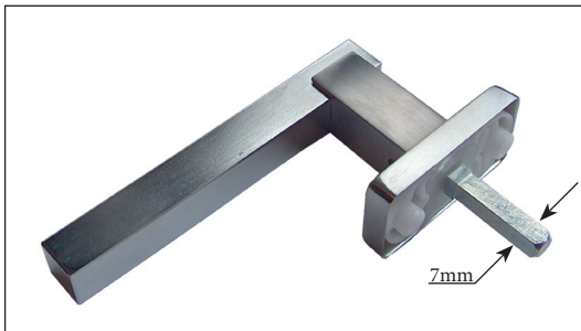
895 CW/350 ΠΟΜΟΛΟ Europa (μικρό) LEVER HANDLE Europa (short)
